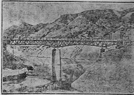
На Военно-Грузинской дороге, в Михте (22 километра от г. Тифлиса) открыт новый мост через реку Куре длиной в 30 метров. Этот мост построен взамен имевшегося, который после пуска ЗАГЭС'а (Село-Амальская гидроэлектрическая станция) должен был быть затоплен водой.
