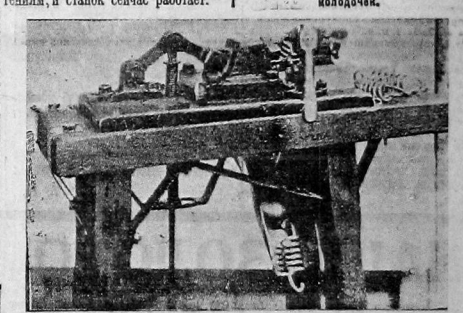
Станок, приспособленный тов. Смирновым для изготовления пружин тормозных колодок.
