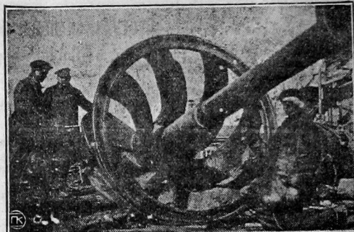
В текущем 1928 году на месте постройки будущей Сиверской гидроэлектрической станции будут производиться экскаваторные и друштвенные работы в канале шлюза силовой станции. На снимке — ремонт разрыхлителя грунта для землесосов Сивазовода
