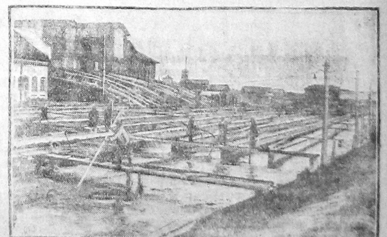
На лесозаводе № 25 в Архангельске построен первый в крае вертикальный отопленный бассейн, на 2 метра выше уровня реки. Подача бревен в бассейн производится элеватором. На снимке: Верхне-молочный отопленный бассейн. Слева — лесозавод.
