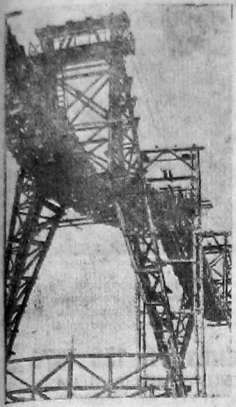
В угольной гавани Одесского порта строится новый 8-мильный перегружатель. Фото Рыбальченко (Союзфото).
