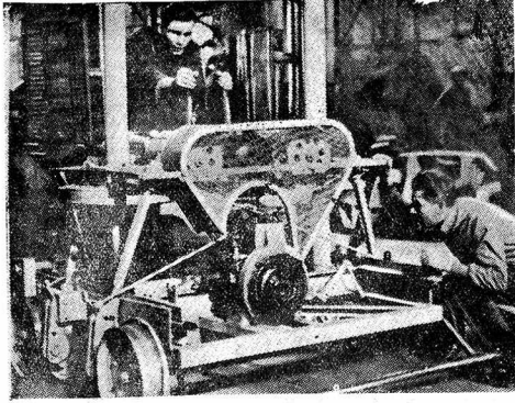
Завод НКПС в Калуге приступил к массовому выпуску вновь освоенных заводом пуделоделинок, дающих возможность одновременно производить подметку пути и смену шпал. На снимке: мастер отделения пуделоделинок В. Р. Старичен (слева) дает готовый пуделоделиник мастеру отдела технического контроля И. К. Маркову (справа).
