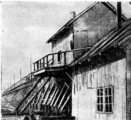
Механизированная эстакада для выгрузки лесоматериалов из реки на Лузской лесопилкостанции треста Севтранлес
