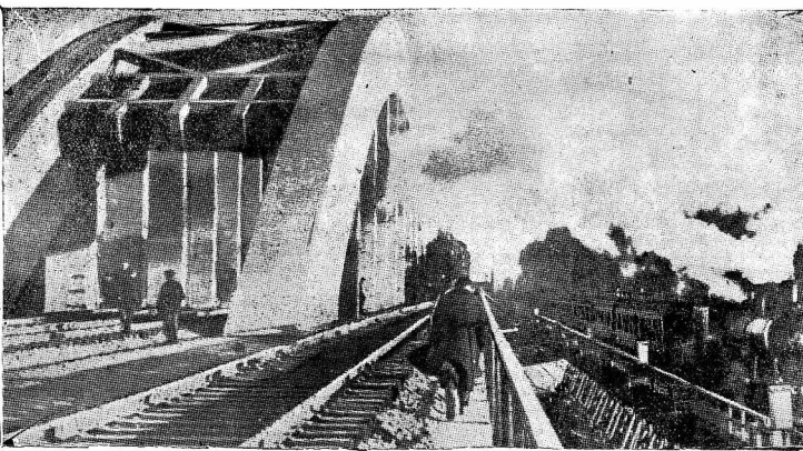
В ноябре комиссия НКПС, возглавляемая тов. Пашковским, проводила испытания нового 4-путного железнодорожного арочного моста через канал Москва—Волга у ст. Хемин Октябрьской железной доро и. По мосту ежедневно проходила 4 паровоза со скоростью 60 километров в час. Испытания дали отличные результаты. На снимке: общий вид нового моста. Фото Вихирева.
