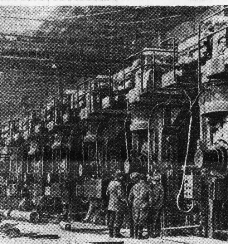
СТАЛИНСКАЯ ОБЛАСТЬ. На Ждановском заводе имени Ильича вступает в строй первая очередь тонколистового стана «1700». Идет последнее опробование механизмов. Фото П. Кашиня. Фотохроника ТАСС.
