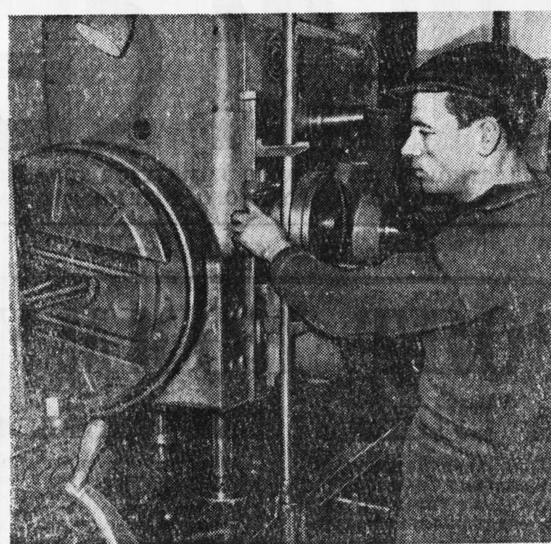
РАСТОЧНИК вологодского завода «Северный коммунар» Алексей Николаевич Козлов выполняет почетный заказ для сельского хозяйства. Он изготовляет коробки передач для тракторов «ДТ-54». Опытный производитель ежедневно обрабатывает по пять коробок передач при норме четыре. На снимке: А. Н. Козлов. Фото А. Жидкова.
