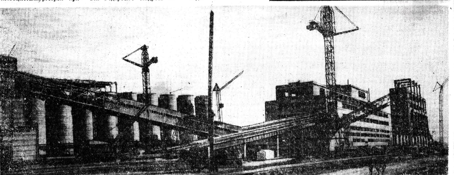
Общий вид на комплекс сооружений углеобработки № 2 Череповецкого металлургического завода.
