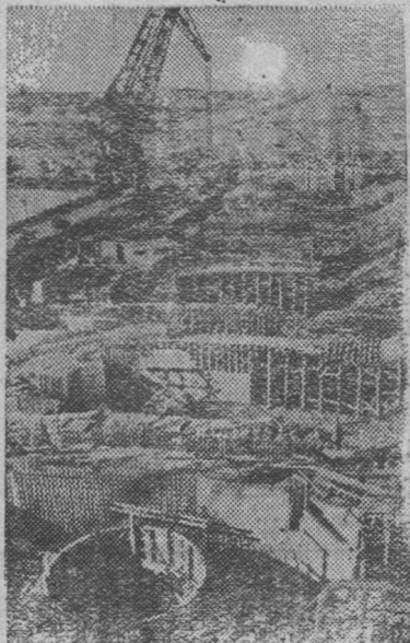
Иркутская область. Недалеко от города Иркутска на реке Ангаре сооружается первая ГЭС Ангарского каскада. Здесь будет установлено 8 гидроагрегатов общей мощностью 660 тысяч киловатт. На всех участках сейчас наблюдается небывалый трудовой подъем. Строители ГЭС готовятся к затоплению котлована и перекрытию русла Ангары. Закачивается укладка бетона в сооружаемую монтажную площадку, на которой будут собираться узлы гидроагрегатов. Два агрегата Иркутской ГЭС в 1956 году дадут первый промышленный ток. На снимке: строительство здания Иркутской ГЭС. Фото П. Лисенкина.
