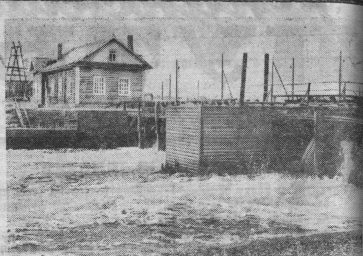
В конце прошлого года на реке Андома была построена и сдана в эксплуатацию межколхозная Князевская ГЭС мощностью 180 киловатт.
