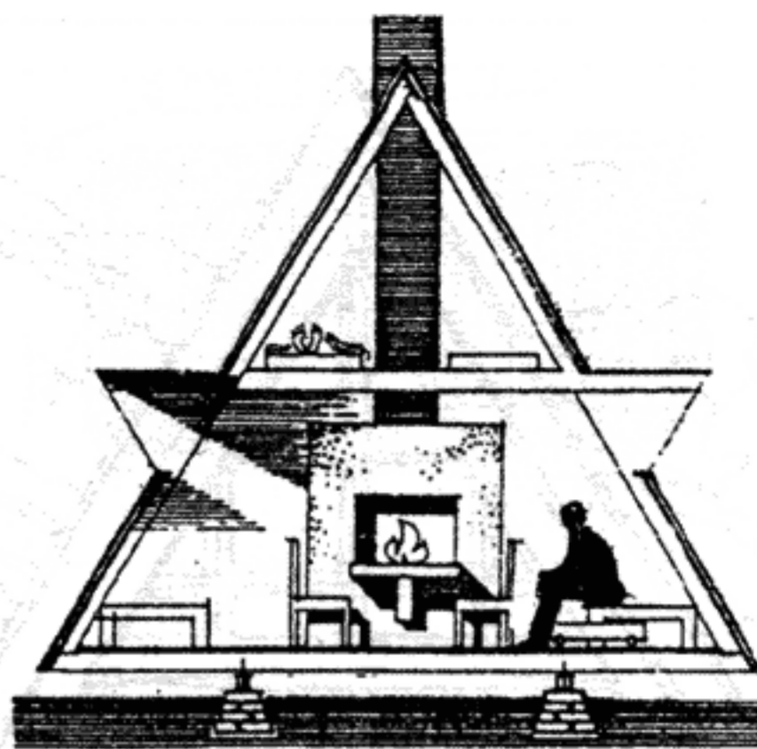
Разрез
