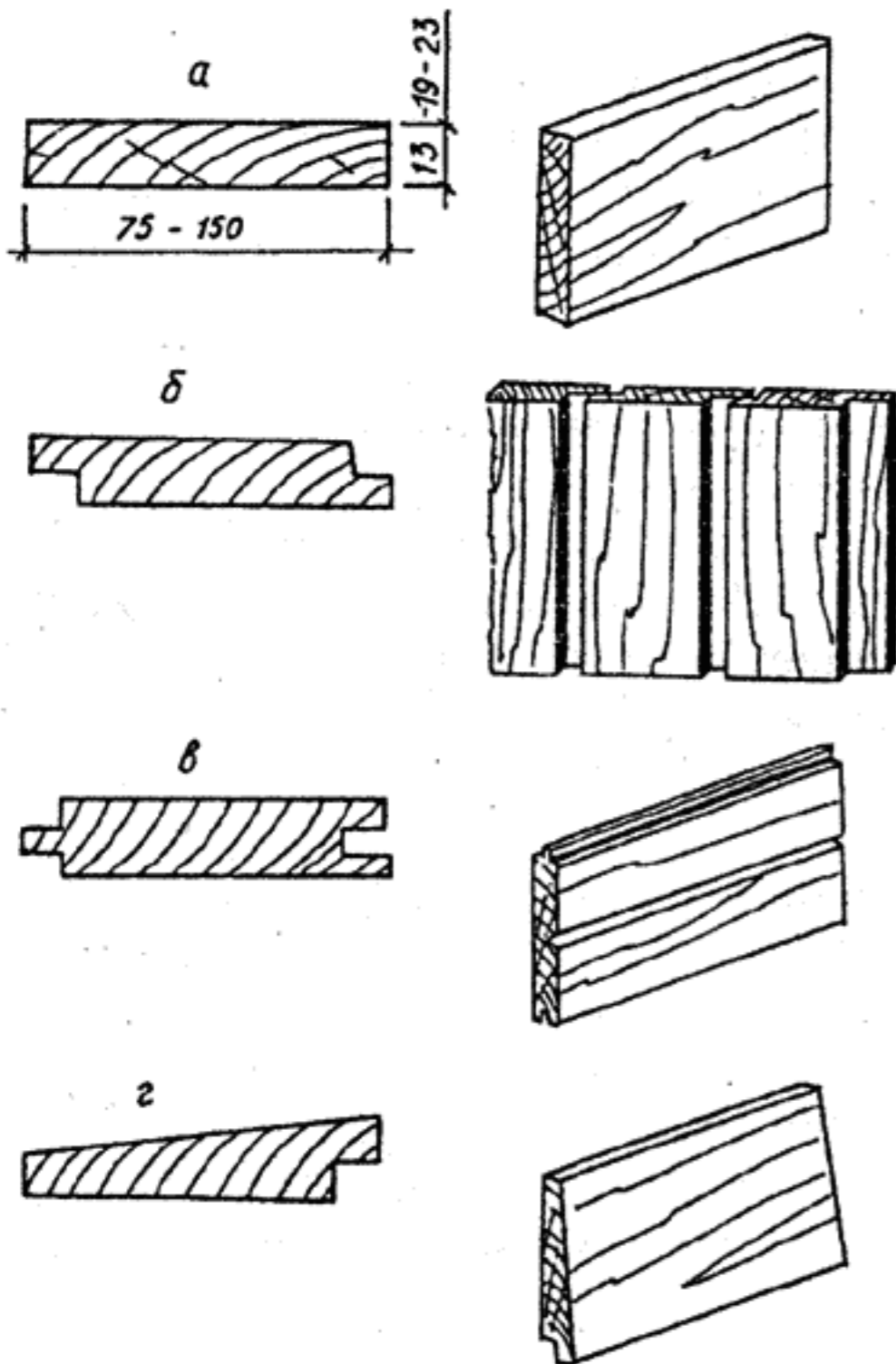
Отделочная доска:
