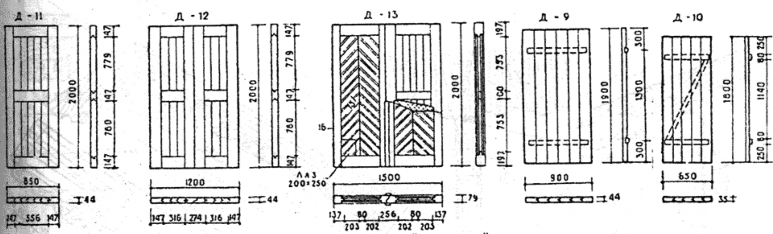
Двери хозяйственной постройки
