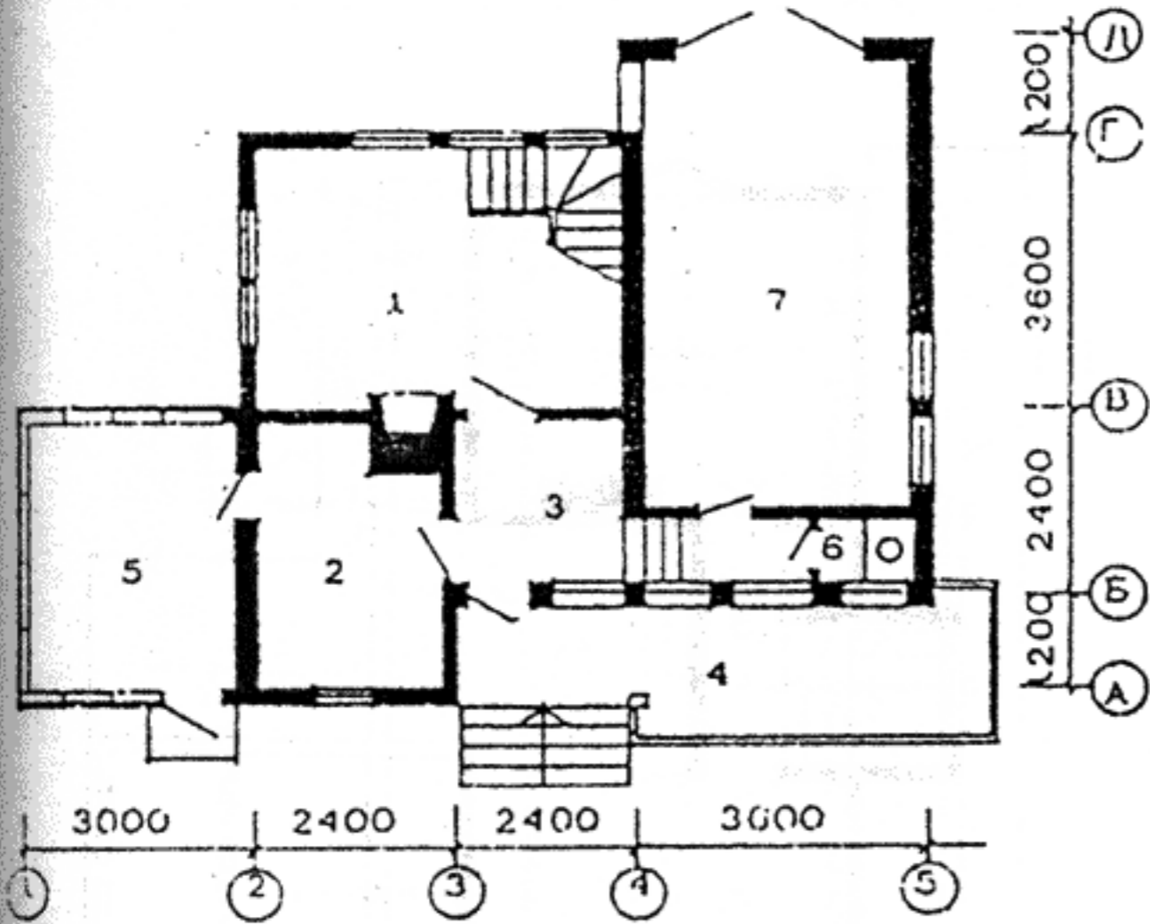
План этажа
