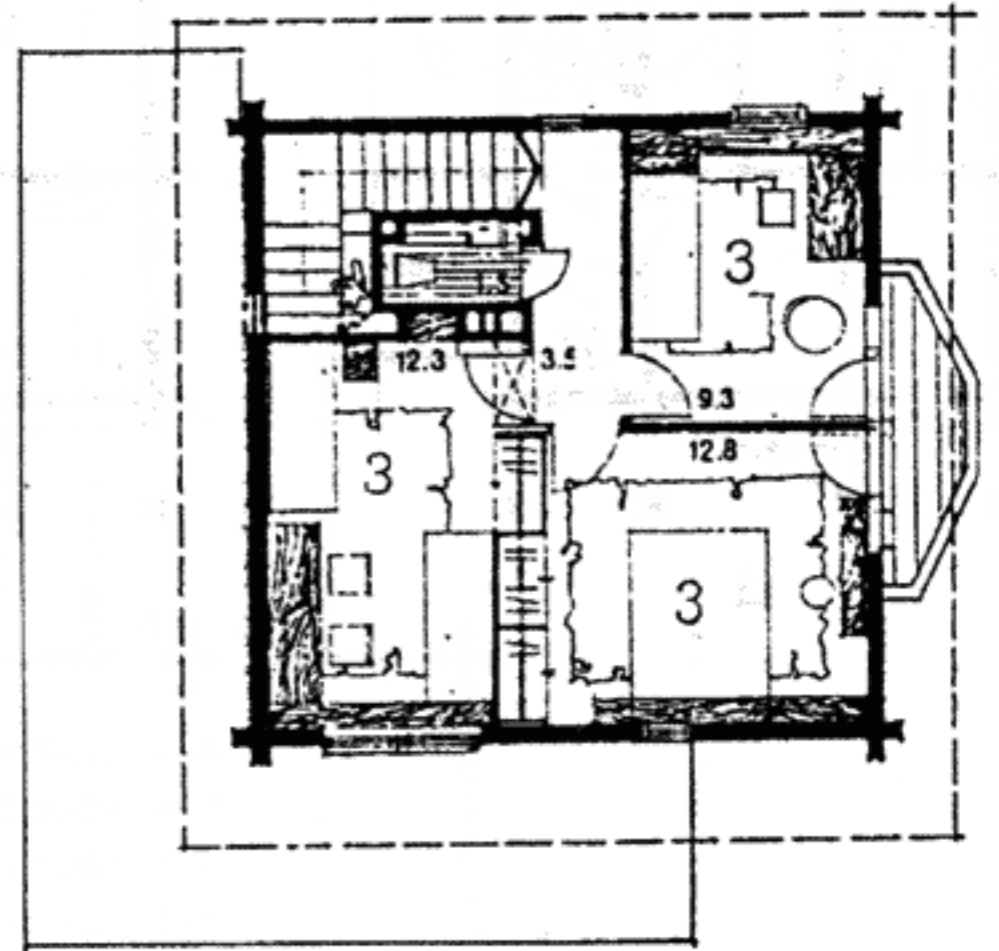
План 2 этажа
