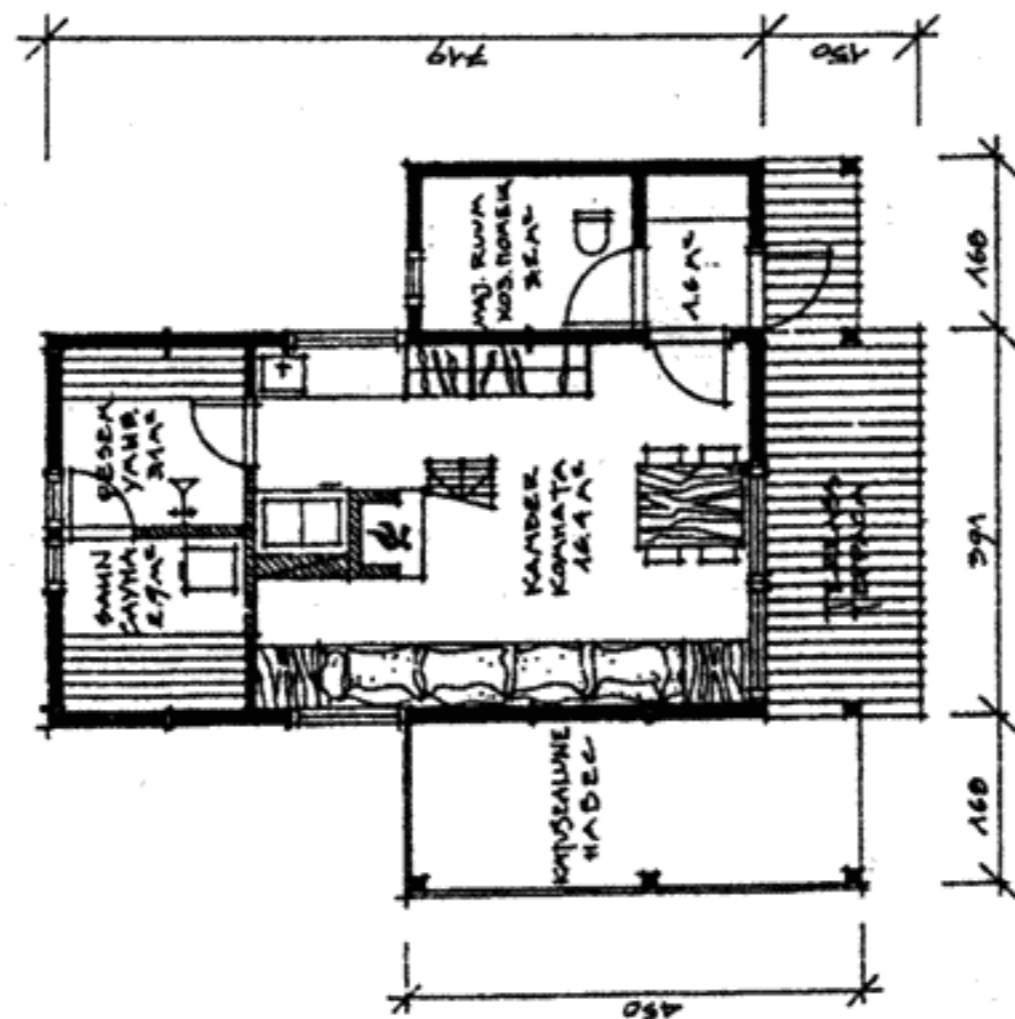
План 1 этажа
