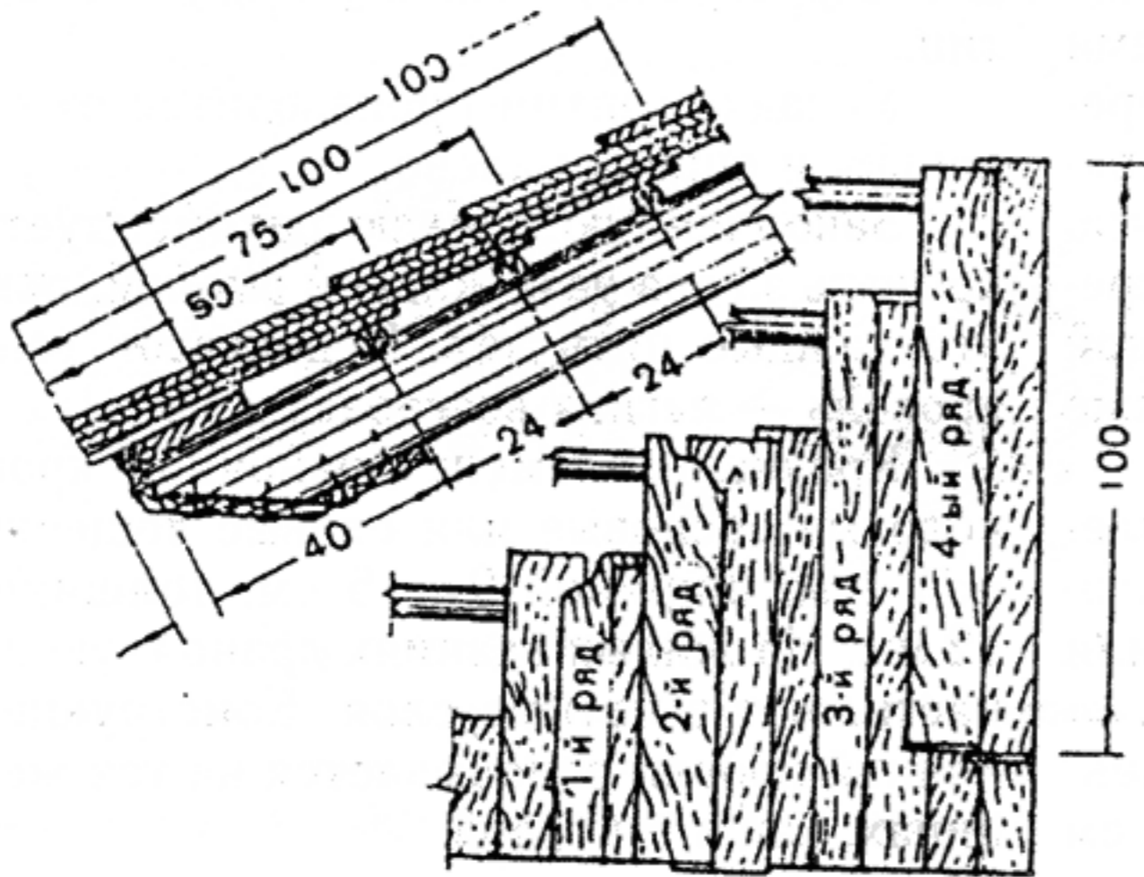
Драничная кровля
