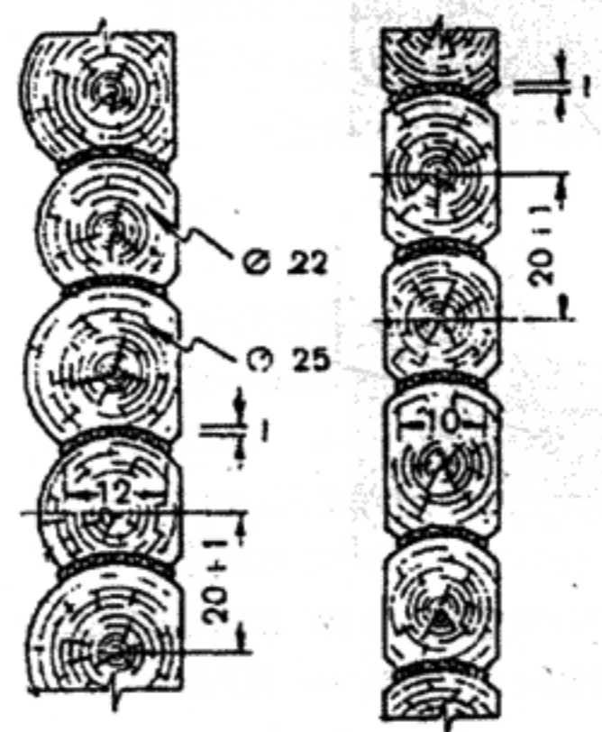
Конструкции бревенчатых стен
