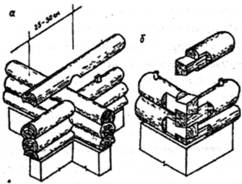
Угол, рубленный в «лапу»
