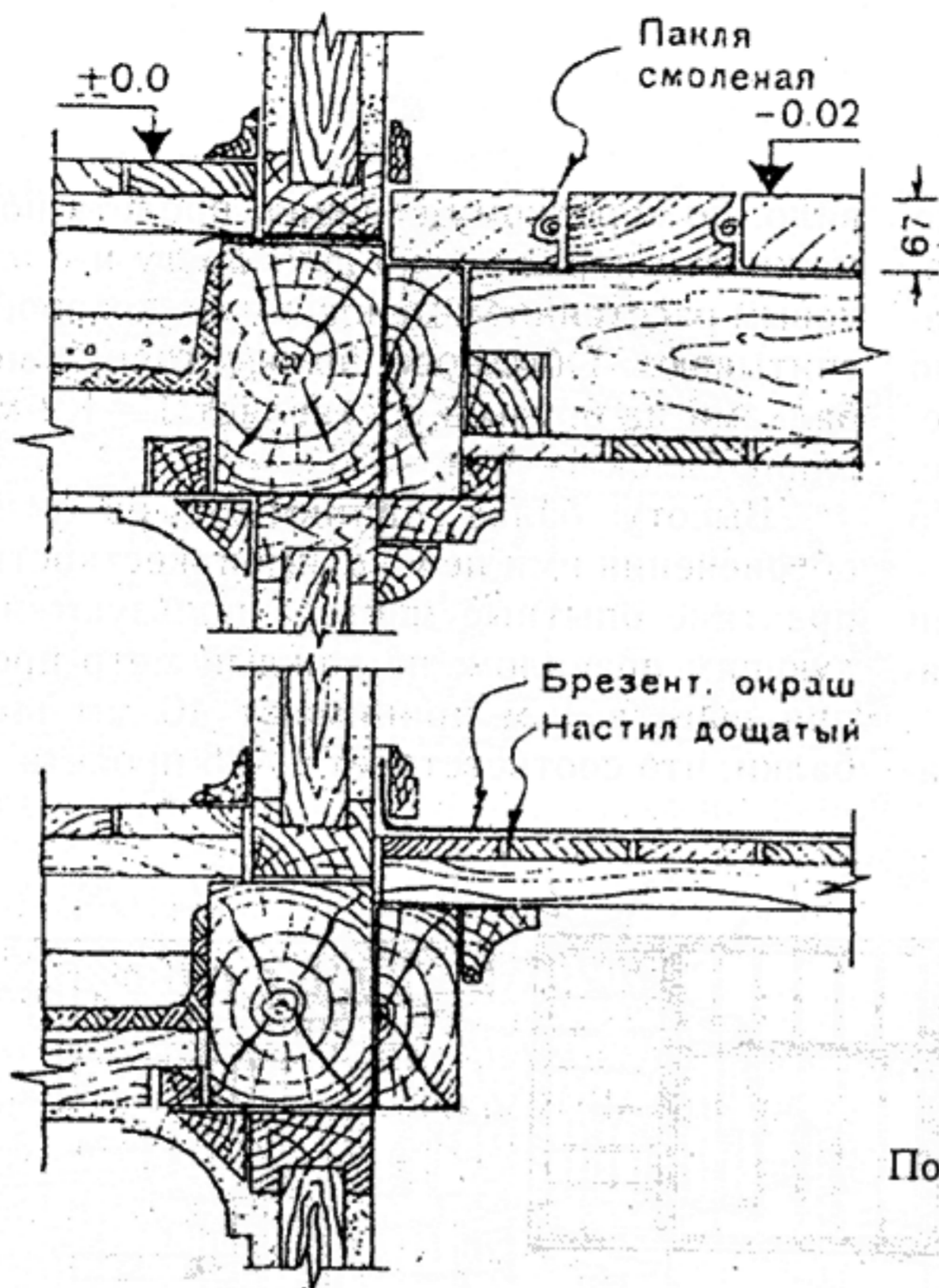
Перекрытия в санитарных узлах
