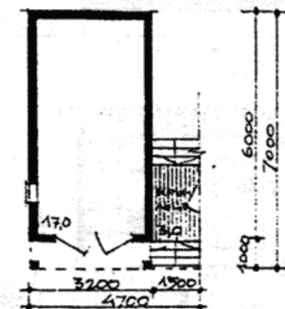
ПЛАН М 1:100
