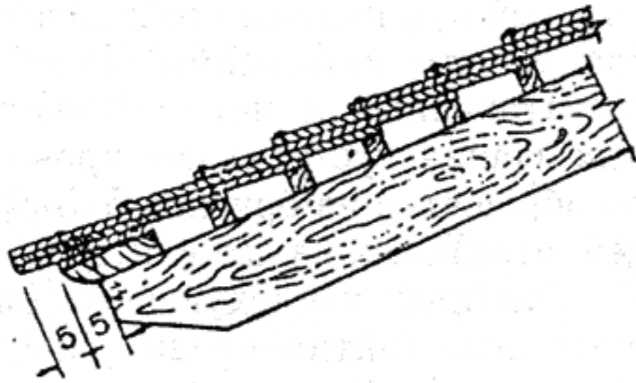
Устройство свеса
