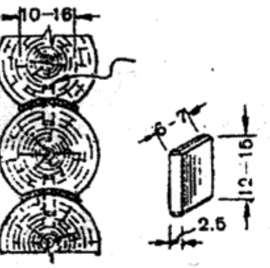
Вставной шип
