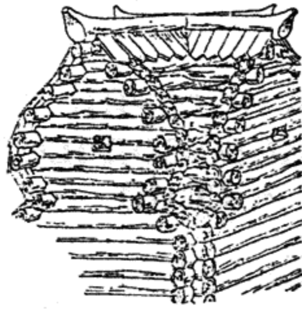
Крестовая бочка
