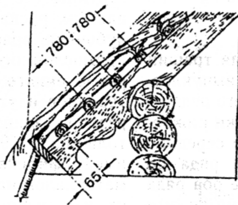
б) разрез
