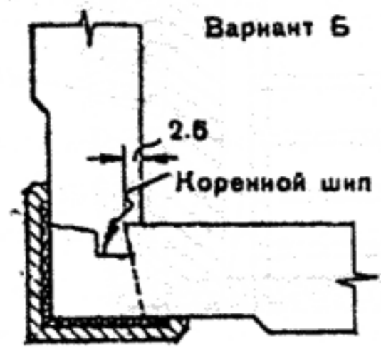
Угол, рубленный в «лапу»
