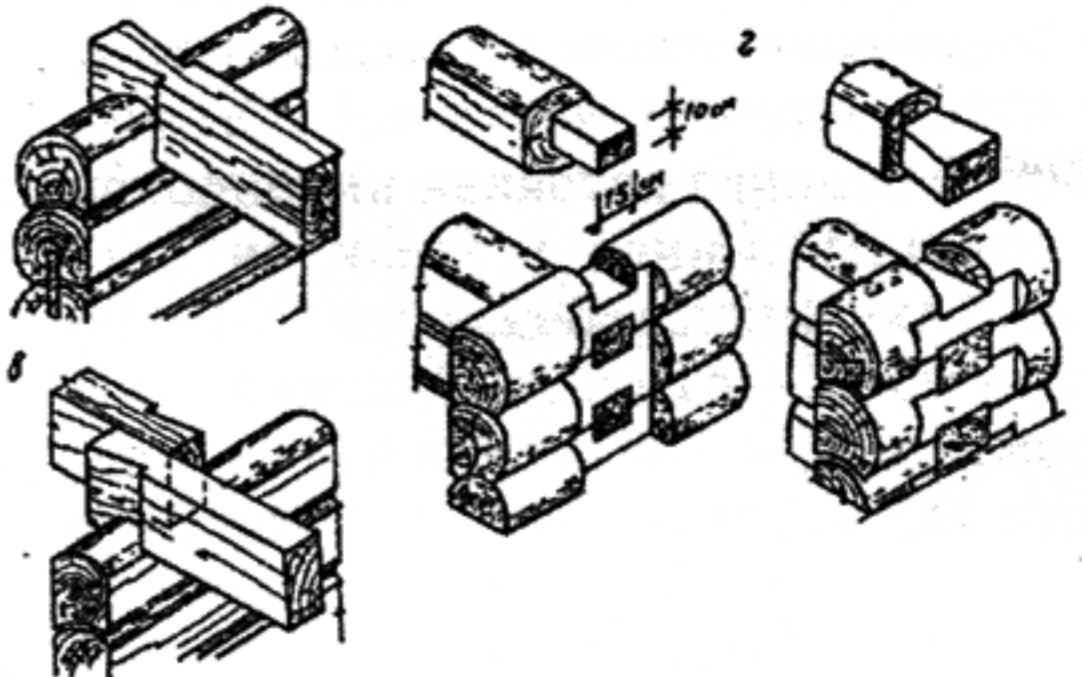
Конструкции бревенчатых стен
