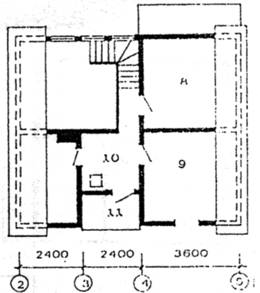
План мансарды
