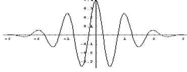
Рис.2. График \mathbf{Re}(G_{0,2\pi}^{0.5}(t)) .
