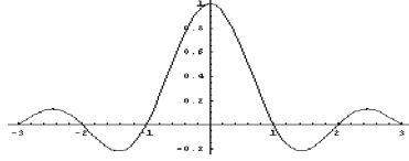
Рис.1. График \varphi^S(t) .
