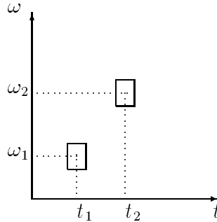
Рис.4. Окна Габора.
