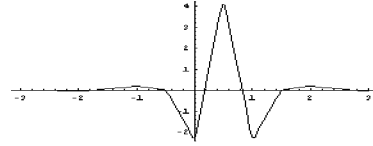
Рис.2. График \psi^{B,2}(t) .
