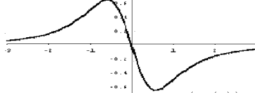
Рис.2. График \mathbf{Im}(\psi(t)) .
