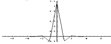
Рис.1. График \varphi^{B,2}(t) .
