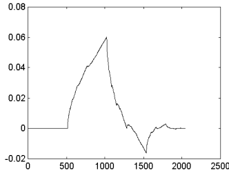
Рис.1. График \varphi^{D,2}(t) .
