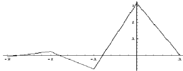
Рис.1. График \varphi^{St,2}(t) .
