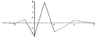
Рис.2. График \psi^{St,2}(t) .
