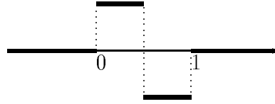
Рис.2. Всплеск Хаара.
