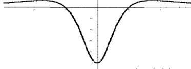
Рис.1. График \mathbf{Re}(\psi(t)) .
