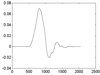
Рис.1. График \varphi^{D,4}(t) .
