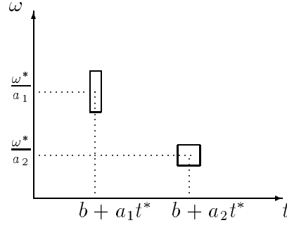
Рис.1. Окна ИВП.
