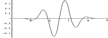
Рис.2. График \psi^3(t) .
