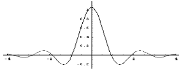
Рис.1. График \varphi^M(t) .
