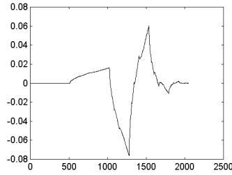
Рис.2. График \psi^{D,2}(t) .
