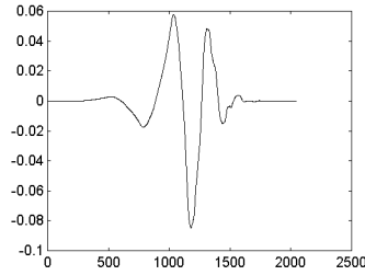
Рис.2. График \psi^{D,4}(t) .
