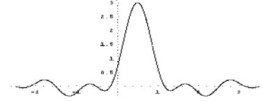
Рис.2. График \psi^S(t) .
