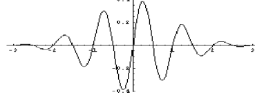
Рис.3. График \mathbf{Im}(G_{0,2\pi}^{0.5}(t)) .
