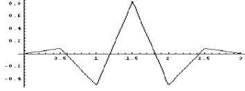
Рис.1. График \psi^2(t) .
