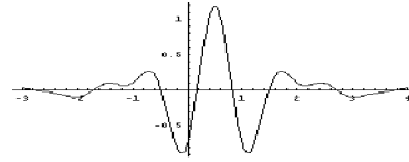
Рис.2. График \psi^M(t) .
