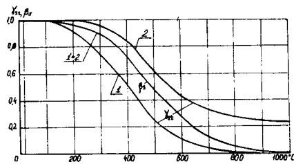
Рис. 4. Значения коэффициентов снижения сопротивления растяжению \gamma_{st} и модуля упругости \beta_s для высокопрочной арматуры класса ВрII
