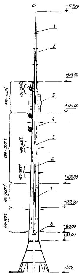
Рис. 1. Схема распространения пожара на телевизионной башне
