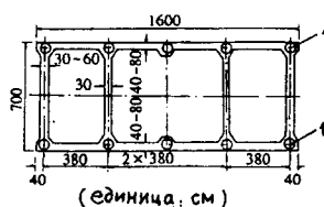
Поперечное сечение арки 1 — трубобетонный пояс
