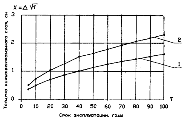
Зависимость глубины карбонизации защитного слоя от срока службы сооружения
