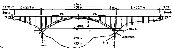
Рис. 7. Схема Ваньсянь моста через р.Янцзы (г.Чунцин)
