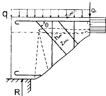
Рис. 3. Наклонное сечение изгибаемого элемента
