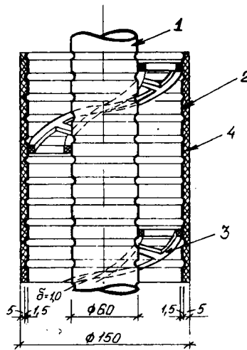
Рис. 2. Высокочастотный фидер
