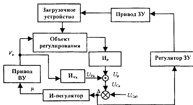
Рис. 1. Структурная схема комбинированной системы управления пневмотранспортированием
