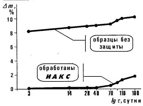
Рис. 2 КИНЕТИКА НАСЫЩЕНИЯ образцов в карналлитовом щёлоче
