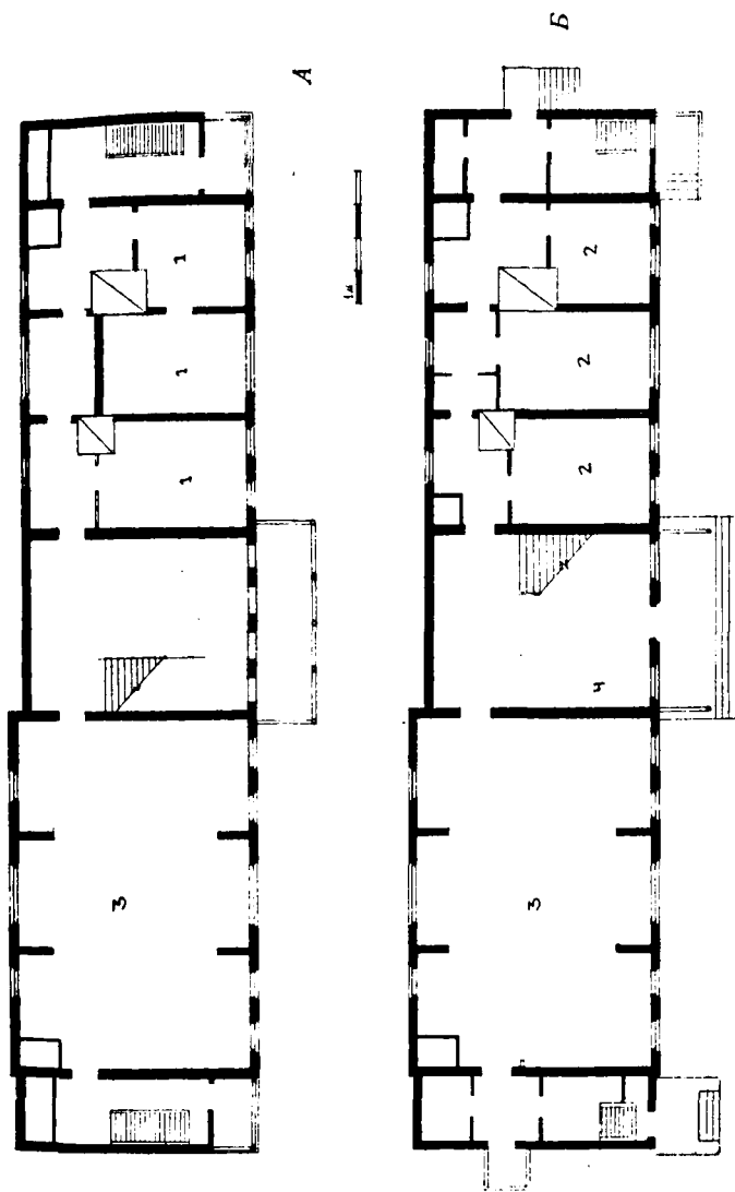
Рис. 2. Волгода. Дом-музей М. И. Ульяновой. А — план второго этажа; Б — план первого этажа.
