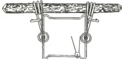
Капкан КП 120 с насторожкой, сдвинутой в сторону
