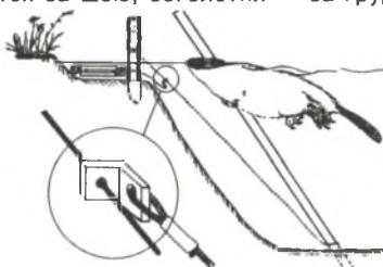
Утапливающая установка капкана № 5
