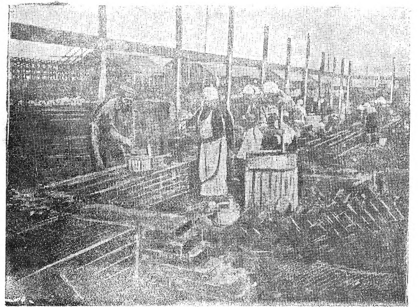
Бригадир Федор Вахрушев с подсобной женской бригадой за кладкой стен гаража Вологодльнострой. Фото Н. ОРЛОВА.
