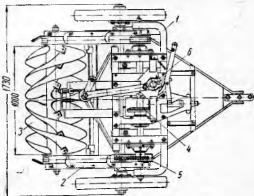
Рис. 2. Схема винтовой фрезы ЛВФС-1:
