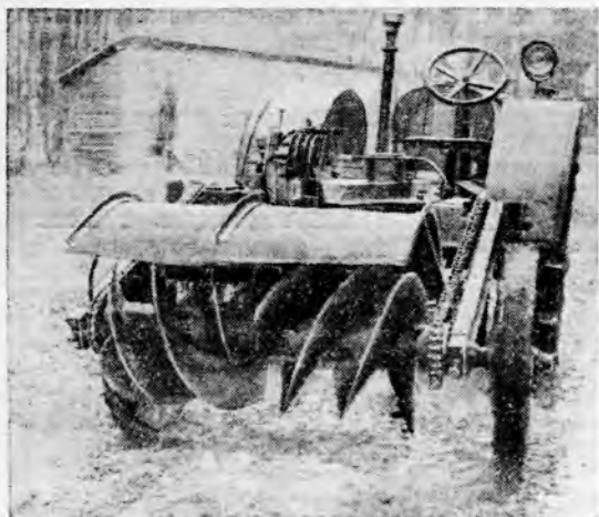
Рис. 1. Винтовая фреза ЛВФС-1
