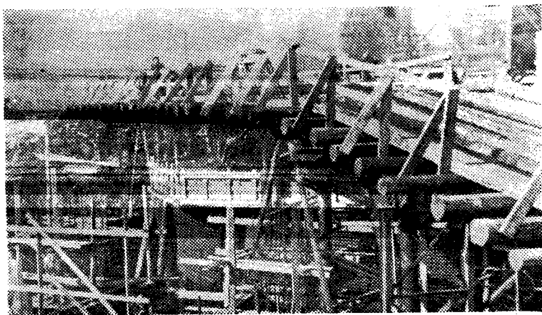
На снимке: вид строительства доменной печи № 4 в г. Череповце. Снимок сделан до начала бетонирования «пня» доменной печи.
