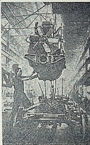
Челябинский тракторный завод. Главный конвейер сборки тракторов С-100.
