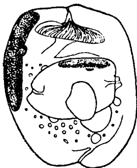
Рис. 2. Entodinium vorax из кожи XXXIII, проглотившей бесшипного Ent. caudatum (650x)
