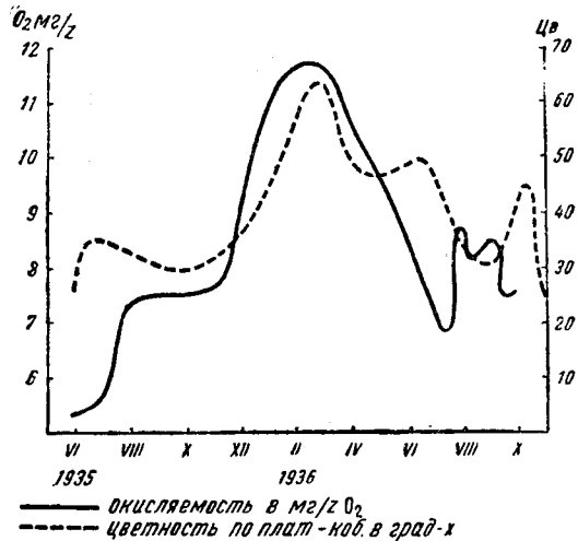
Рис. 5. Цветность в градусах и окисляемость в мг/ O_2 на метр поверхности водохранилища
