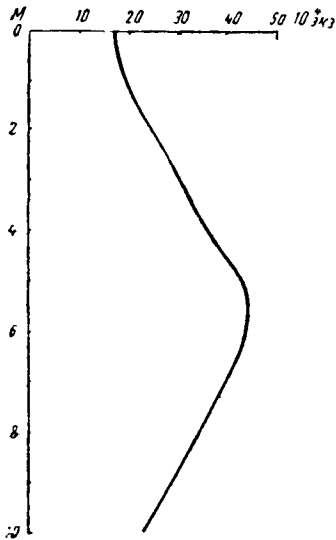
Рис. 7. Вертикальное распределение планктонических организмов 24 сент. 1936 г.
